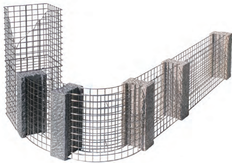
石柱 1~3段(埋込タイプ) 端柱・中柱・コーナー柱
